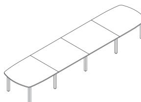
BUN27 5600 / 1300 / 740 305 kg
