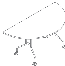
PFT07 800 / 1600 / 740 31.3 kg
