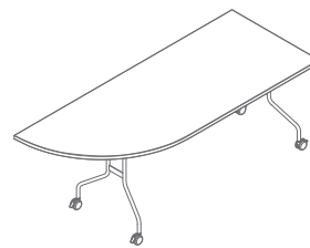
PFT04 2000 / 800 / 740 41.3 kg
